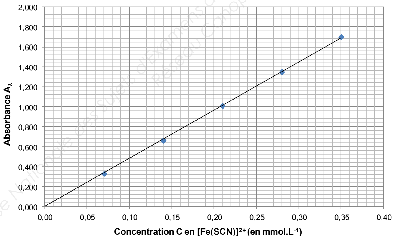
Absorbance d'une solution de complexe [\text{Fe}(\text{SCN})]^{2+}_{(\text{aq})} en fonction de sa concentration, réalisée à une longueur \lambda = 480 \text{ nm} (courbe d'étalonnage)
